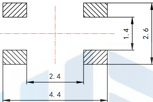
PCB. 焊接图
