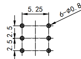
PCB参考图
