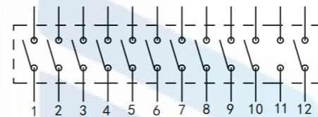
电路图
