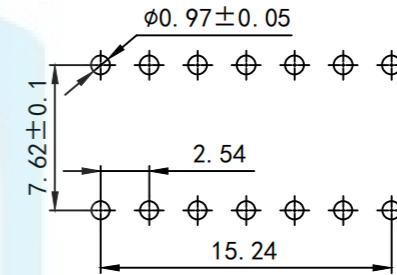
PCB开孔
