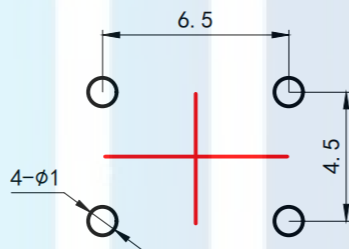
PCB. 焊接图
