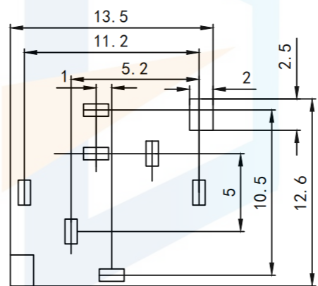
线路板安装尺寸示意图
